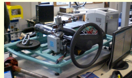
Direction assistée électrique
