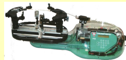
Cordeuse automatisée de Raquette
